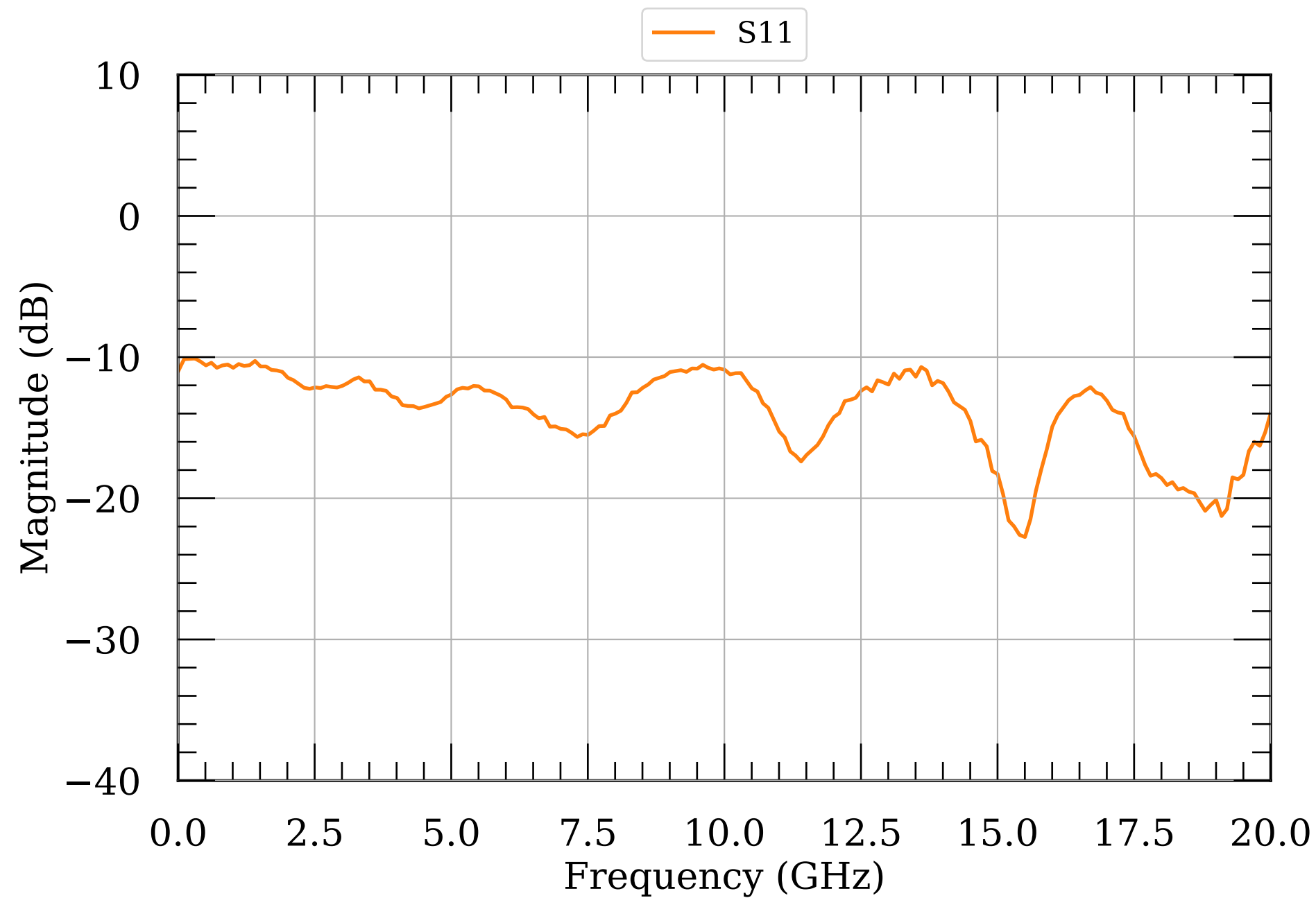
LNA S-params module057
